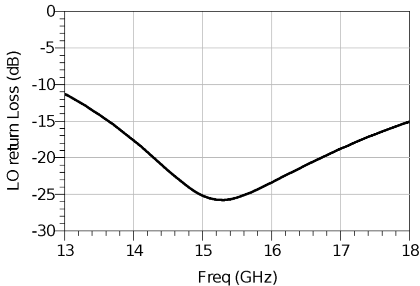
LO Port Return Loss
